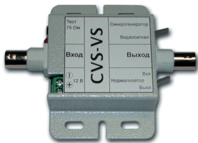
Рис. 3. Анализатор видеосигнала - видеоскоп
