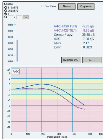
Рис. 2а. АЧХ IP камеры
