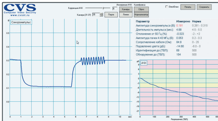
Рис. 4. Видеосигнал. Витая пара 300 м
